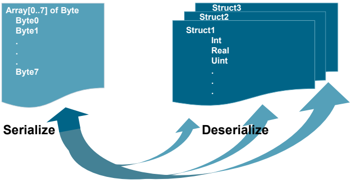
图 2 -30: Serialize 和 Deserialize（S7-1500 和 S7-1200 FW4.1 或更高版本）
