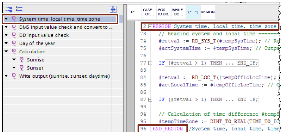
图 3 -56: SCL 编辑器
