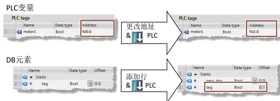
图 2 -40: 更改地址或添加行
