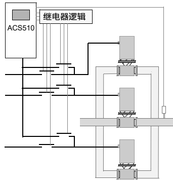
带自动切换的PFC模式
