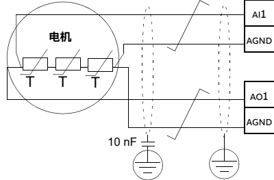
三个传感器
