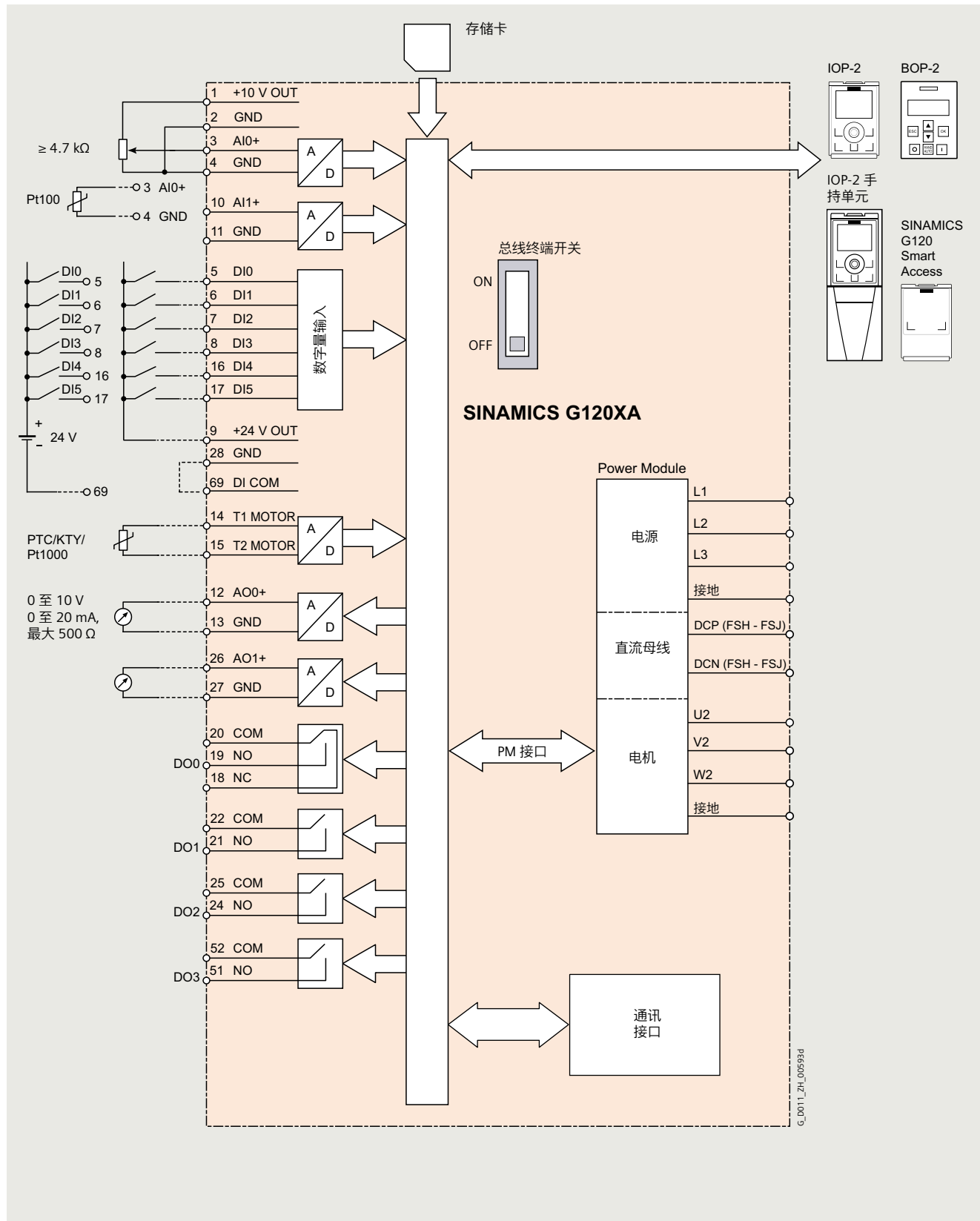
SINAMICS G120XA 接线图, 带控制单元, USS、Modbus RTU、BACnet MS/TP 版
